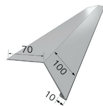
9. Lietskardė, maža | 70/100 mm
