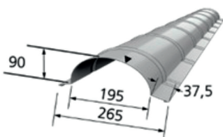
5. Apvalus kraigas | Elegant
