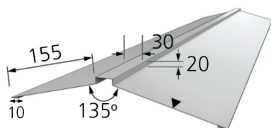
1. Ventiliacinis kraigas, didelis
