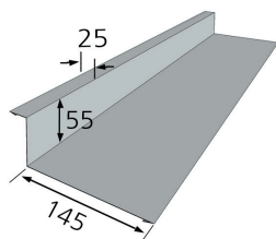
13. Jungtis su siena, šoninė | Classic
