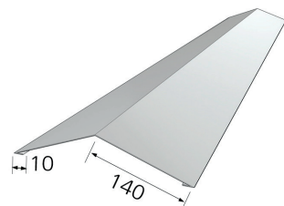
4. Trikampis kraigas, mažas
