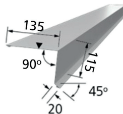
6. Plati vėjaskardė | 135/115 mm
