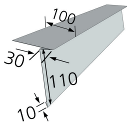
10. Lietskardė | Classic (užkabinama)
