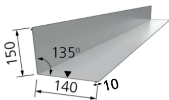
11. Jungtis su siena | 150/140 mm
