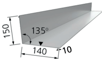
12. Jungtis su siena, galinė | Classic
