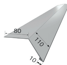
8. Lietskardė, didelė | 80/110 mm
