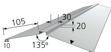
2. Ventiliacinis kraigas, mažas
