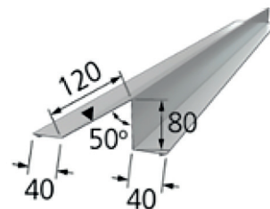
14. Sniego užtvara, didelė | 120/80 mm
